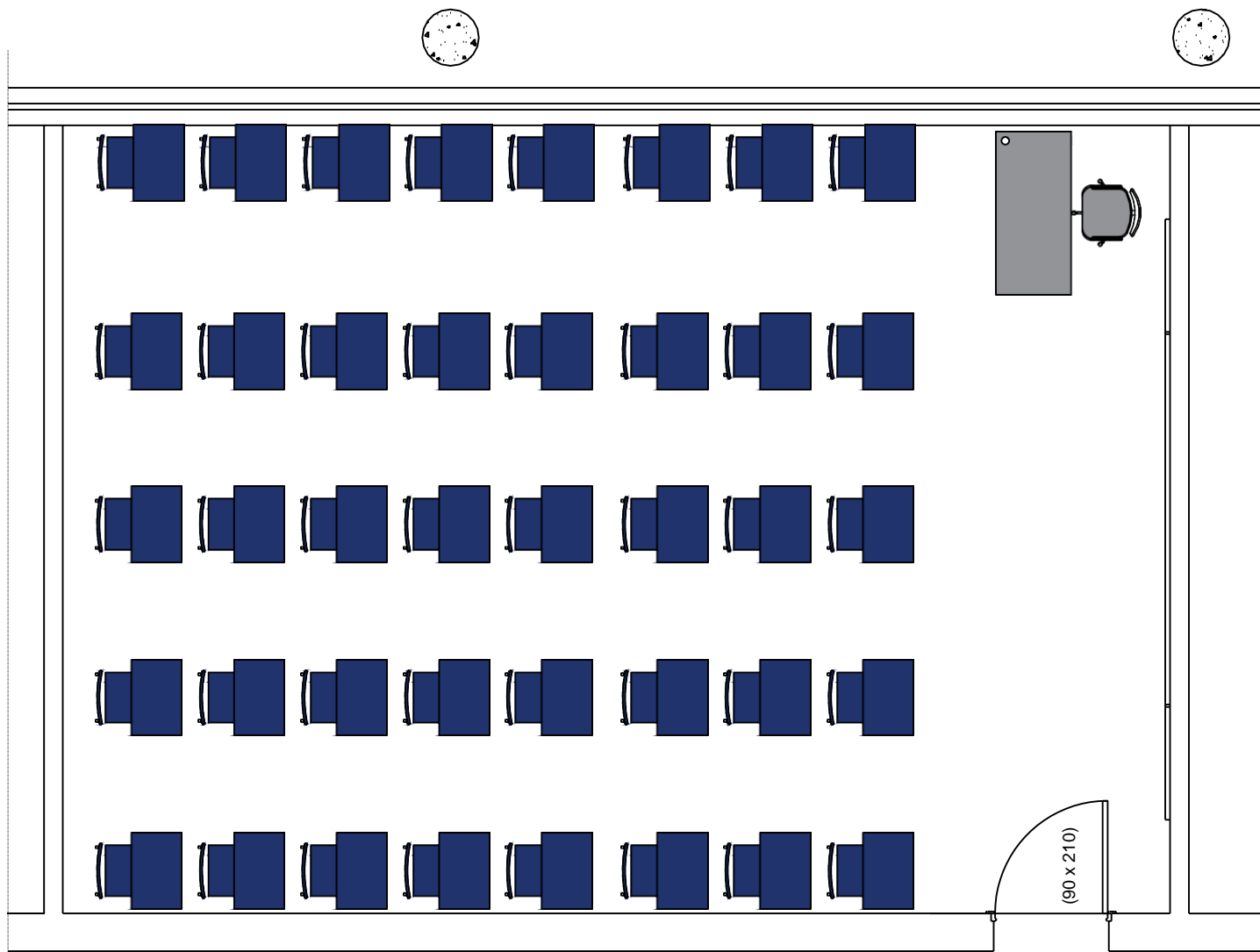
PLANTA DE LAY-OUT ESCALA: 1:50 SALA PADRÃO 40 ALUNOS
