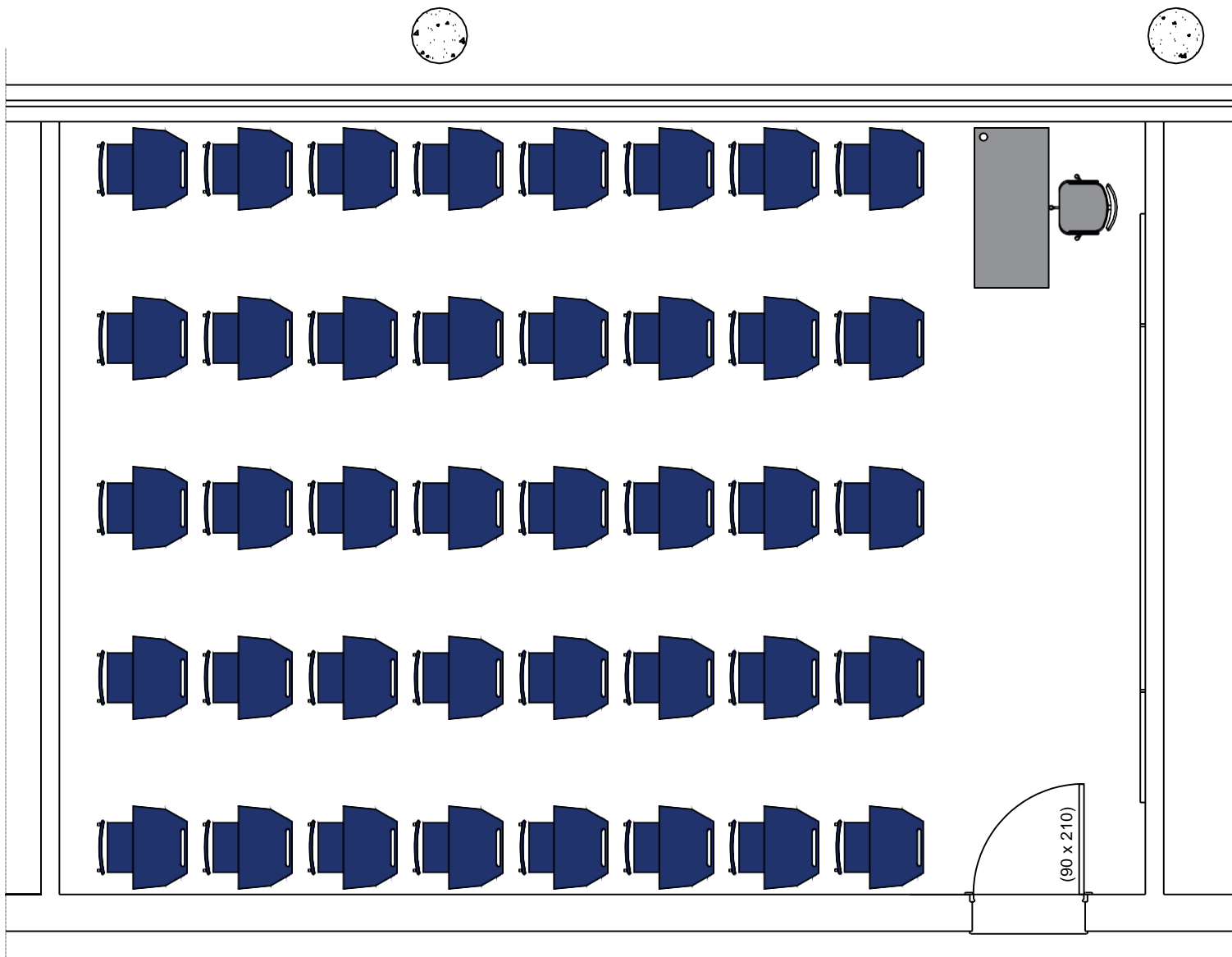
PLANTA DE LAY-OUT ESCALA: 1:50 SALA PADRÃO 40 ALUNOS
